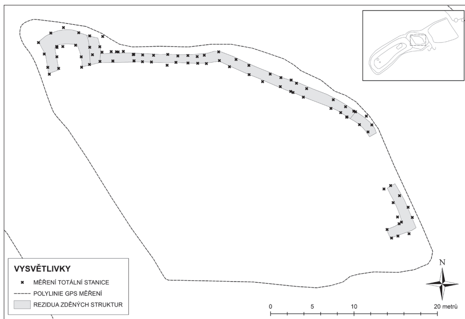
Obr. 2. Hrad Vildenberk (okr. Brno-venkov). Plán předhradí se zaměřením nové objevených úseků obvodové hradby. Zaměření R. Bíško, J. Nedbalová, M. Hlavica a J. Kovář, vizualizace M. Hlavica.
