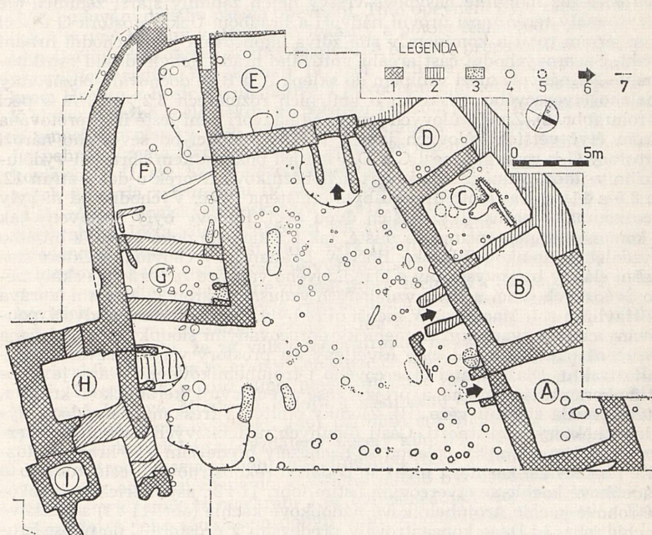
Obr. 2. Lelekovice-Hrad. Celkový plán prozkoumané plochy vnitřního hradu v letech 1984—1989. A, B, C, D — severozápadní palácový trakt, E — velký sklep, F, G — jihovýchodní trakt, H — vysunutá věž, I — brána ve vnějším opevnění. Legenda: 1 — dochované zdivo, 2 — zdivo v negativu, 3 — propálení, 4 — kúlová jamka, 5 — nejasné zahloubení, 6 — vstup, 7 — hranice výzkumu. Kresba: J. Unger—P. Opatřil.
