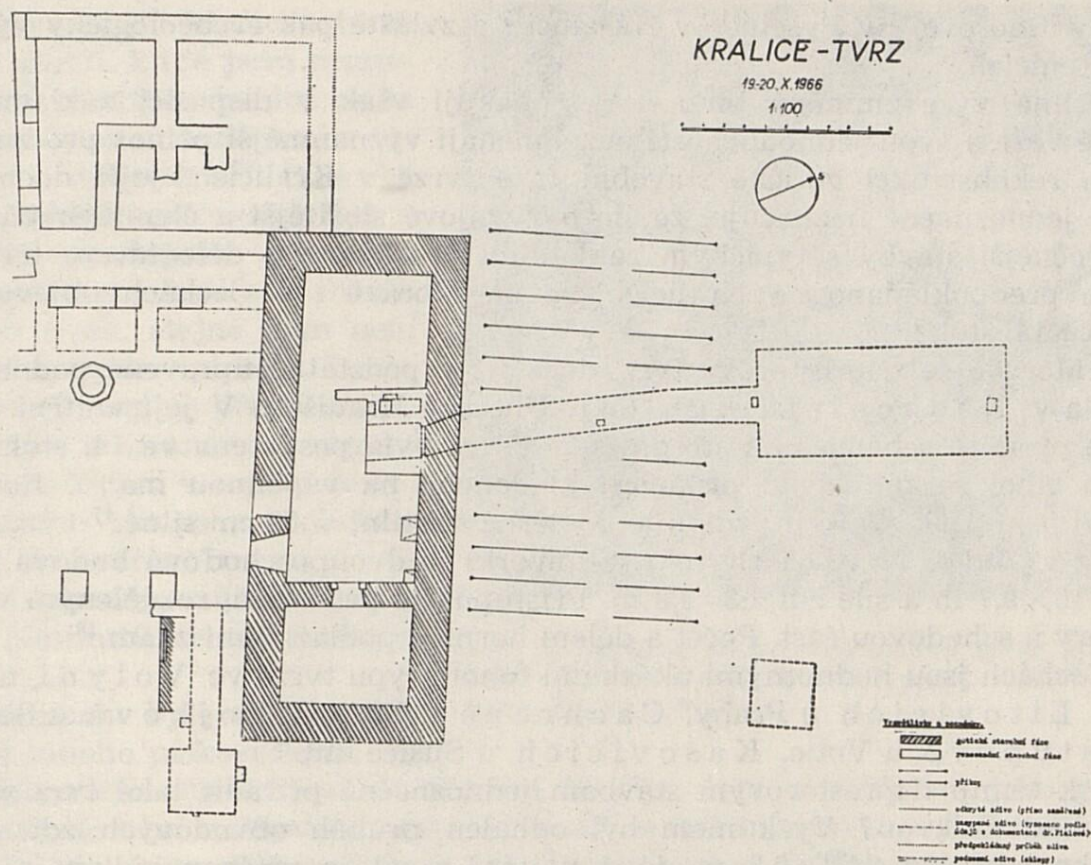
Obr. 1. Archeologickým výzkumem zjištěné části tvrze. Podle Vlasty Fialové. Šrafovaná plocha = gotická fáze; ostatní = renesanční fáze; nepřerušené čáry = odkryté a změřené zdivo; čerchované čáry = zasypané zdivo vynesené dle písemných poznámek V. Fialové; tečkované čáry = předpokládaný průběh zdiva; čárkované = podzemní objekty, tj. sklepy. Polygon na nádvoří = studně. Vyznačení sklonu = příkop.
