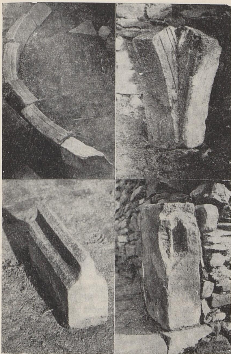
Obr. 4. Vykopané architektonické články. 1 — oblouk arkády, 2 — rohový fragment archivoly, 3 — klenební žebro, 4 — špaleta dveřního otvoru.
