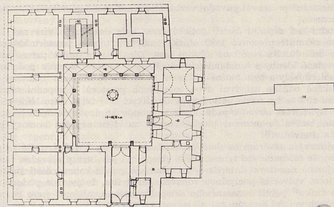
Obr. 1. Archeologickým výzkumem zjištěné části tvrze. Podle Vlasty Fialové. Šrafovaná plocha = gotická fáze; ostatní = renesanční fáze; nepřerušené čáry = odkryté a změřené zdivo; čerchované čáry = zasypané zdivo vynesené dle písemných poznámek V. Fialové; tečkované čáry = předpokládaný průběh zdiva; čárkované = podzemní objekty, tj. sklepy. Polygon na nádvoří = studně. Vyznačení sklonu = příkop.
